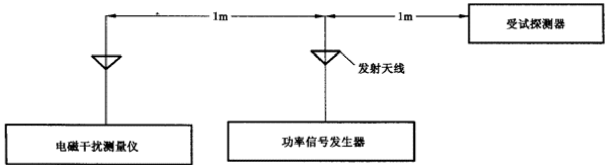
图 1 试验设备布置图
