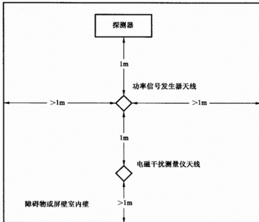
图 2 天线位置图
