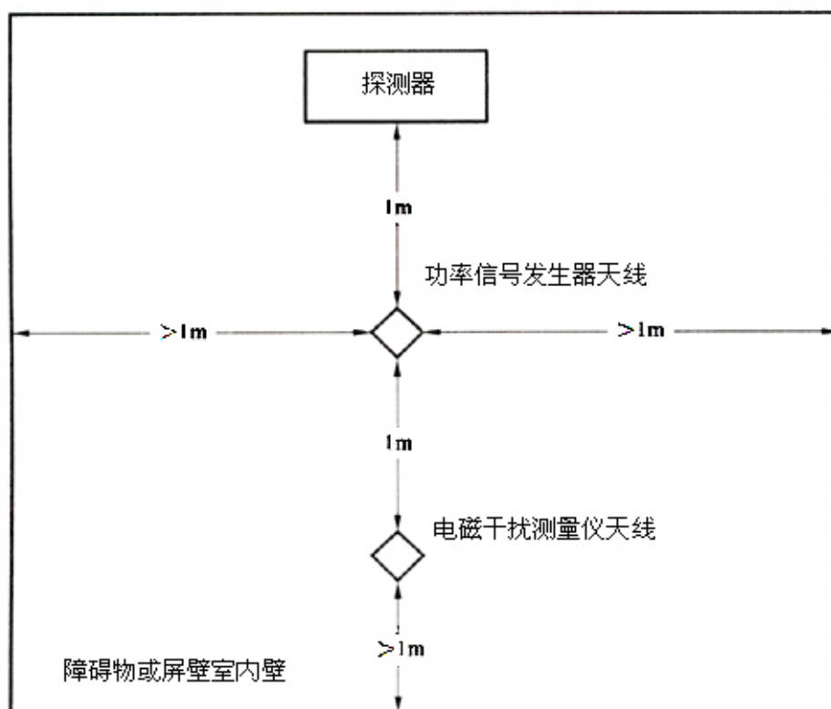
图 2 天线位置图
