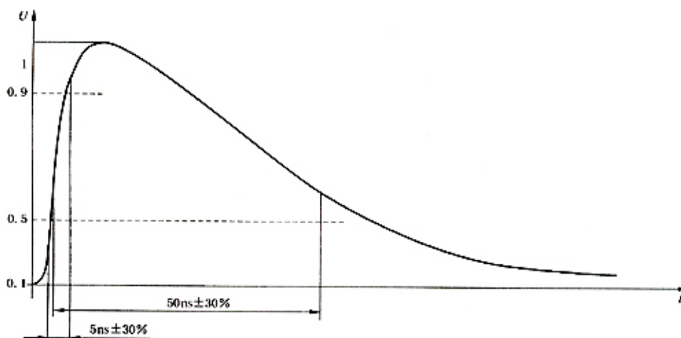
图 3 50Ω 负载时单脉冲波形
