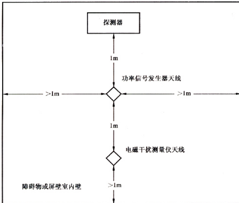
图 2 天线位置图
