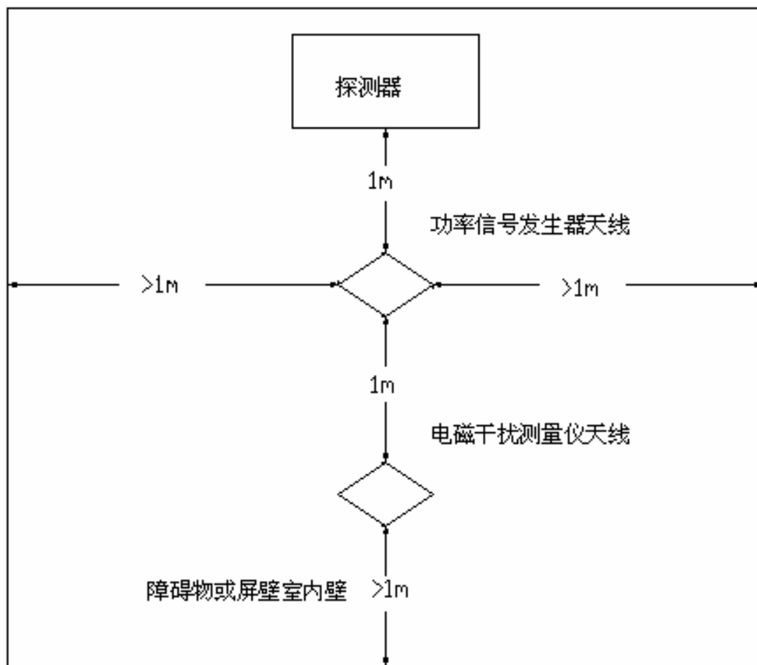
图 2 天线位置图
